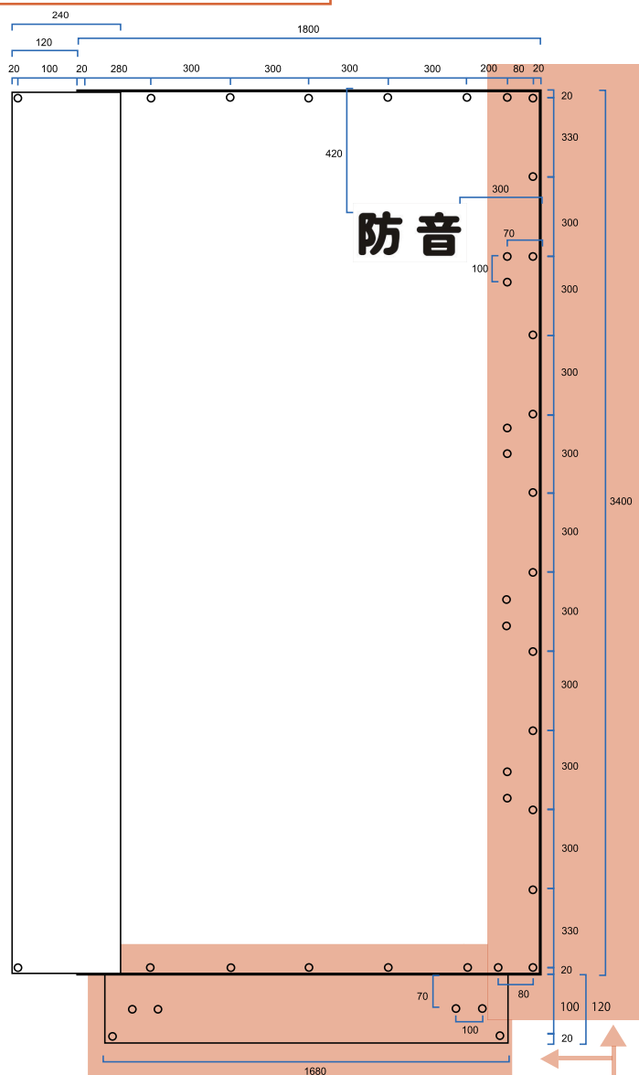
防音シート R型裏面 1.8×3.4m 図面
